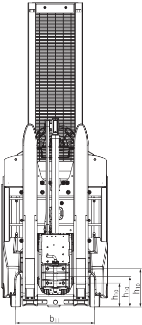
Vista trasera con horquillas plegadas
