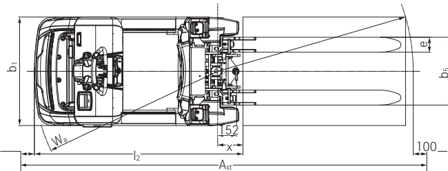
Vista superior
