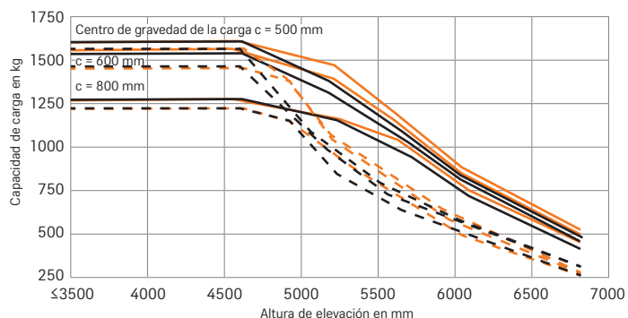
RXE 16C Mástil triple - ruedas SE sencillas 180/70-8, Ancho de 990 mm + 1028 mm
